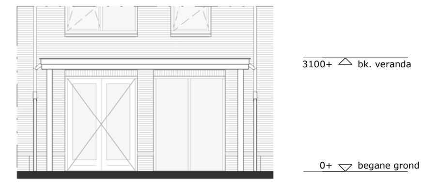
achtergevel - 1 : 100
