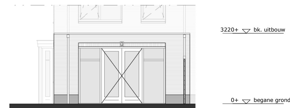
achtergevel - 1 : 100
