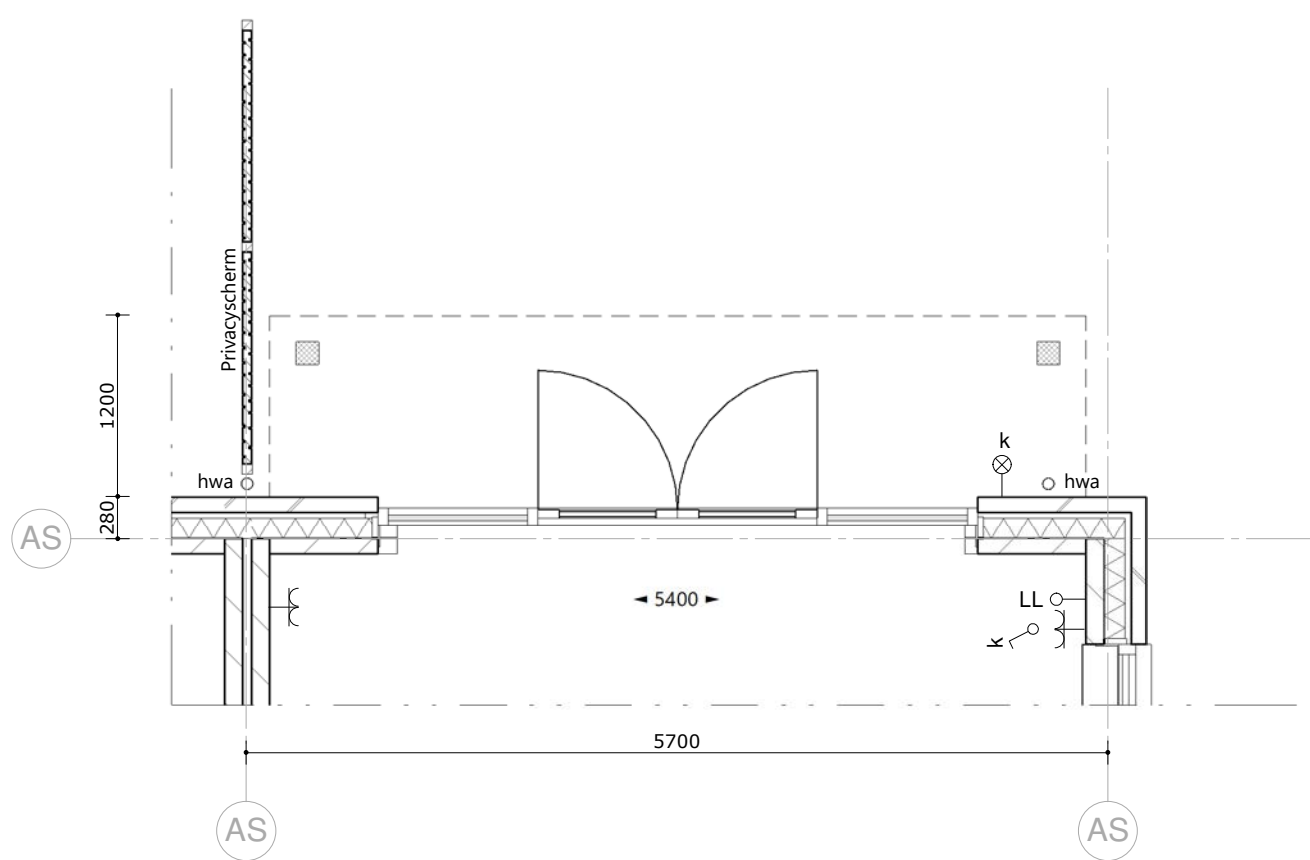
begane grond - 1 : 50
