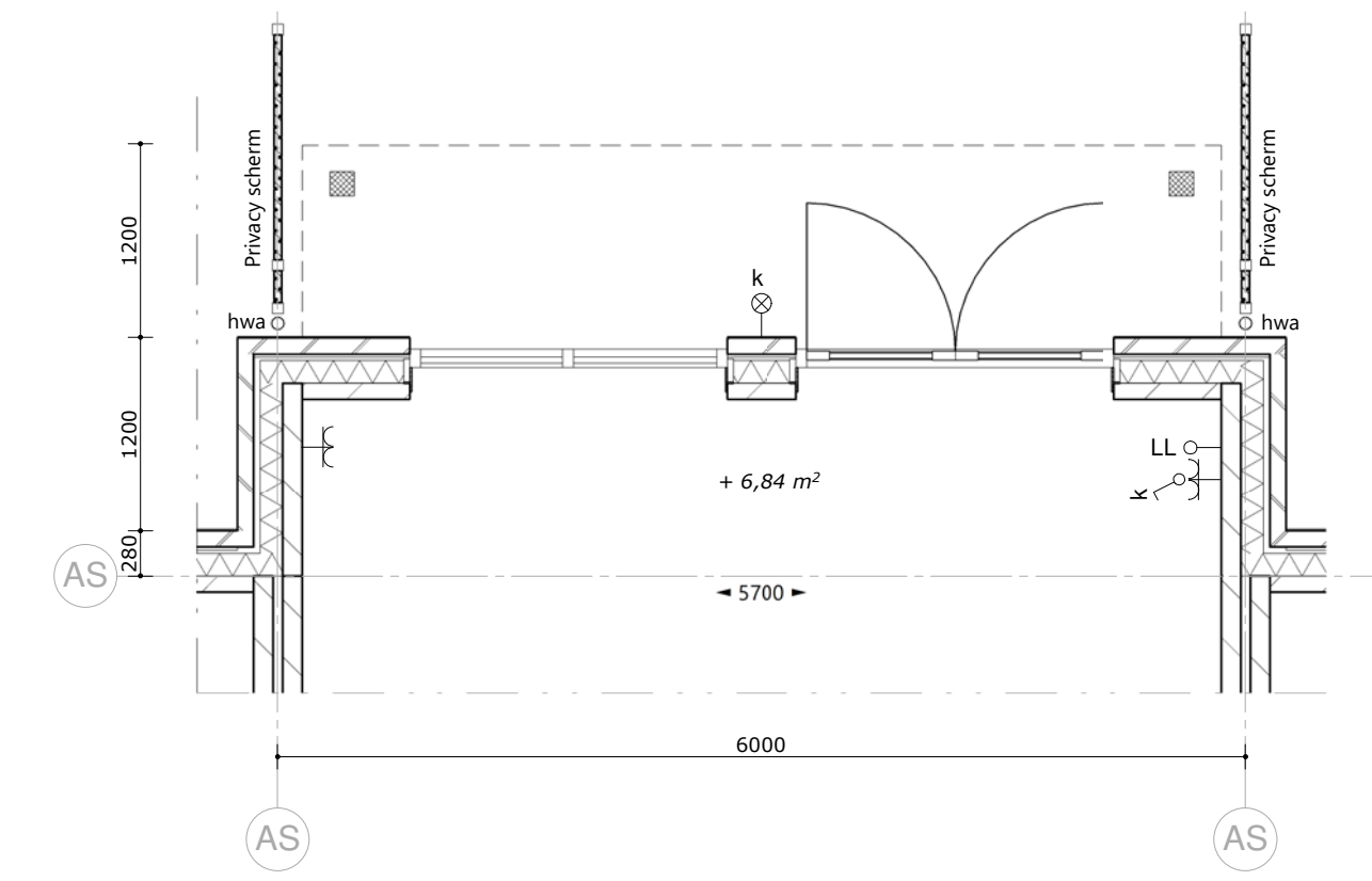
begane grond - 1 : 50
