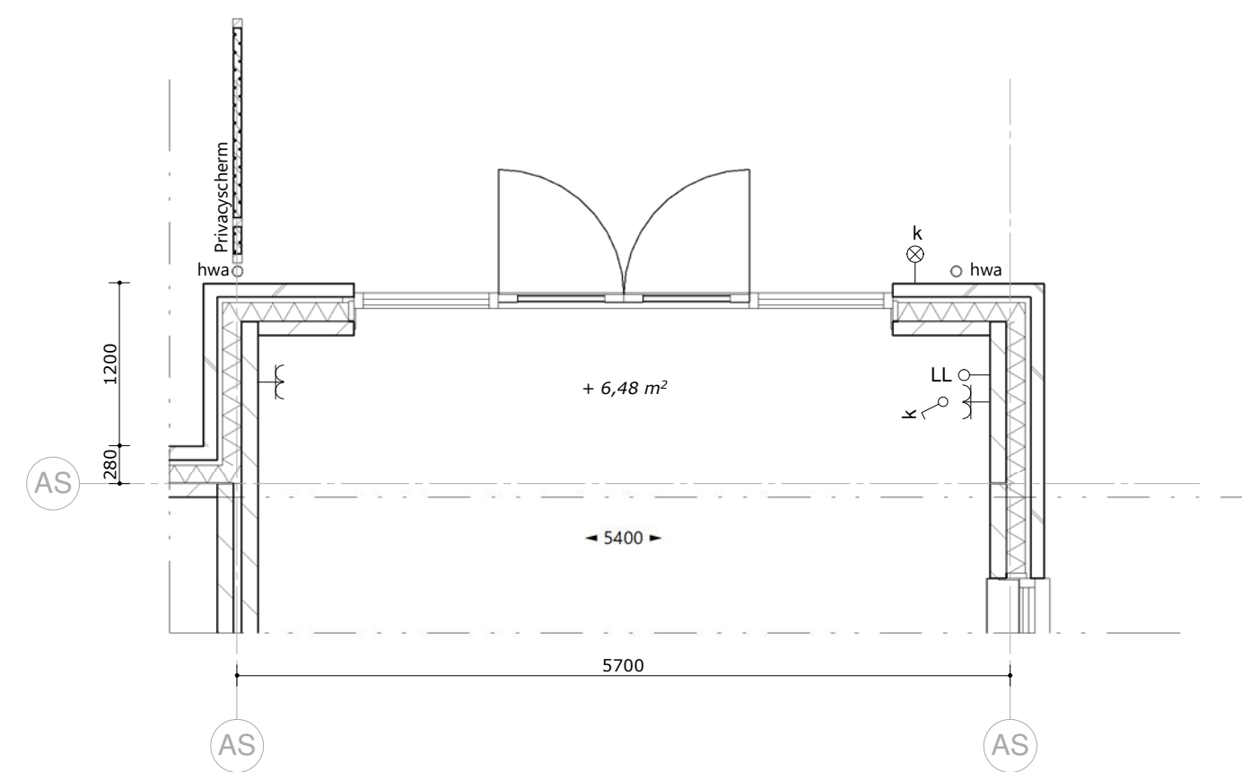
begane grond - 1 : 50
