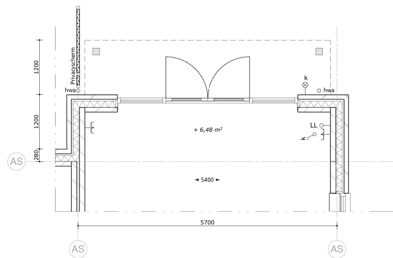
begane grond - 1 : 50
