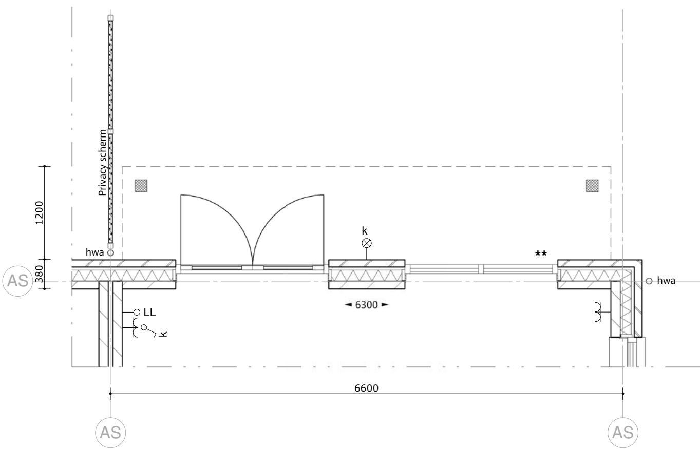
begane grond - 1 : 50
