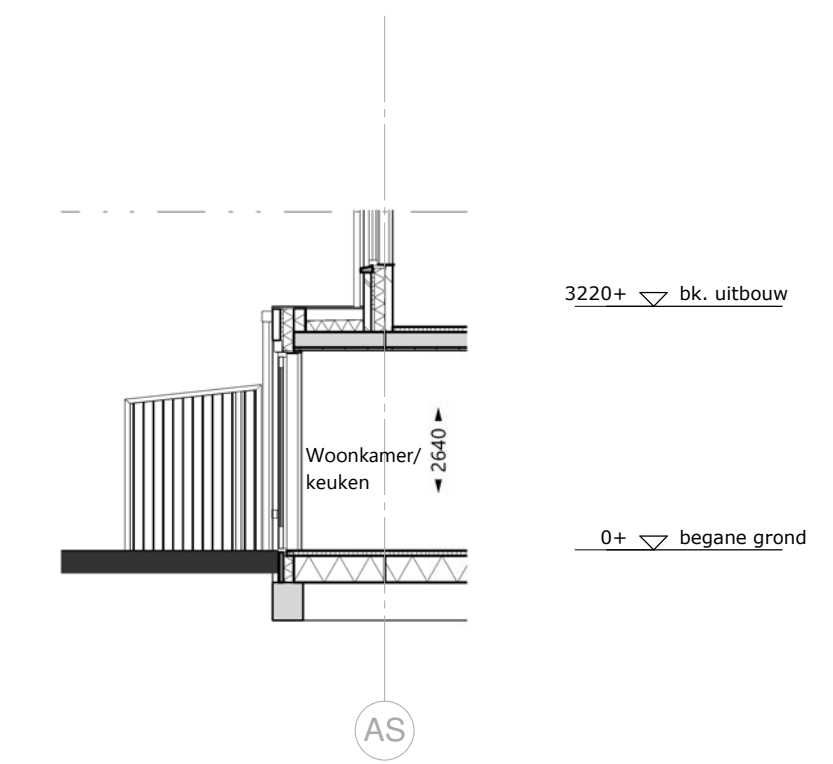
doorsnede 1-1 - 1 : 100
