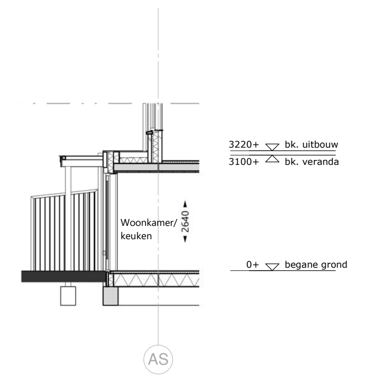
doorsnede 1-1 - 1 : 100
