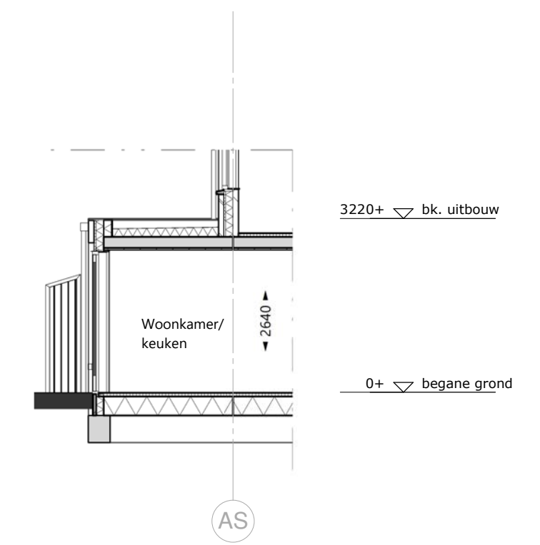
doorsnede 1-1 - 1 : 100
