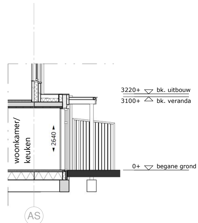
doorsnede 1-1 - 1 : 100
