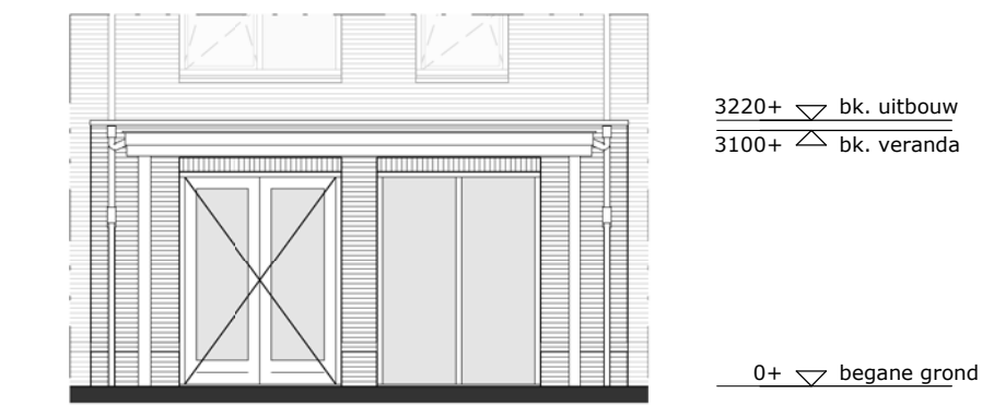
achtergevel - 1 : 100
