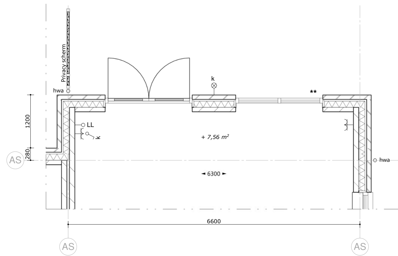
begane grond - 1 : 50
