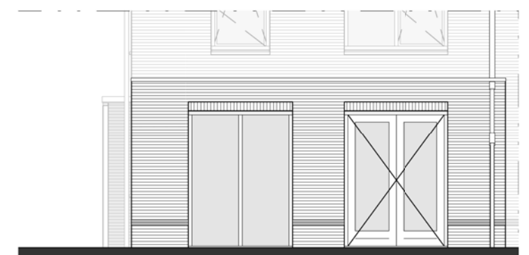
achtergevel - 1 : 100
