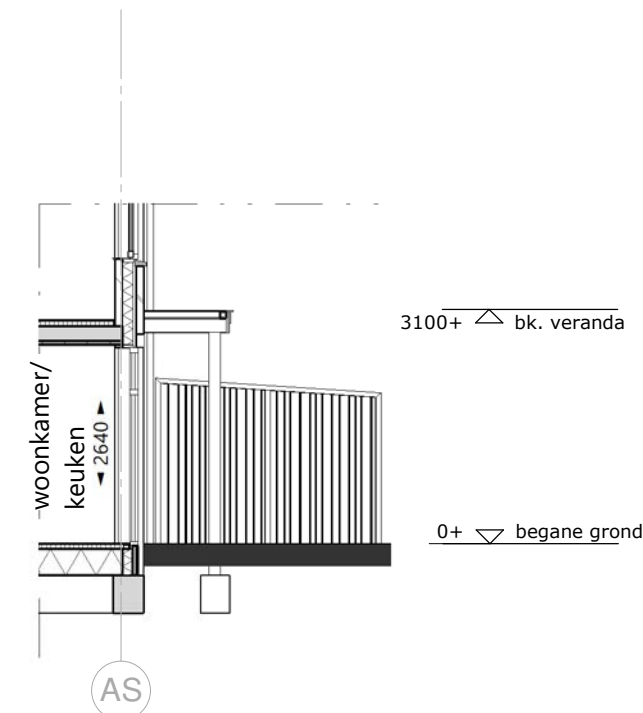
doorsnede 1-1 - 1 : 100
