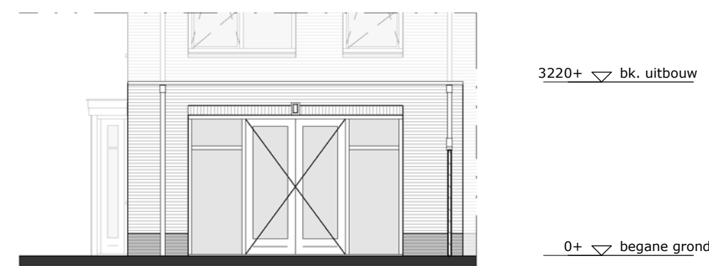
achtergevel - 1 : 100
