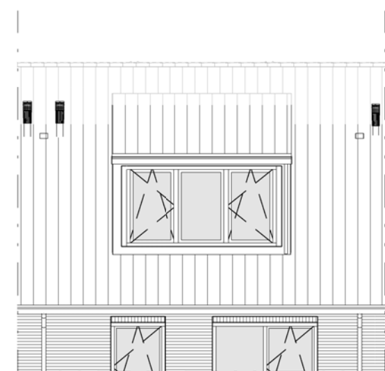
achtergevel - 1 : 100
