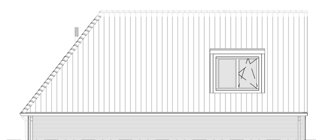
linkergevel - 1 : 100
