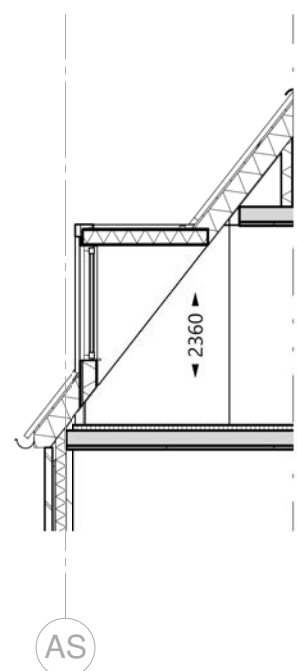
doorsnede 1-1 - 1 : 100
