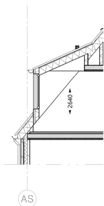
doorsnede 1-1 - 1 : 100
