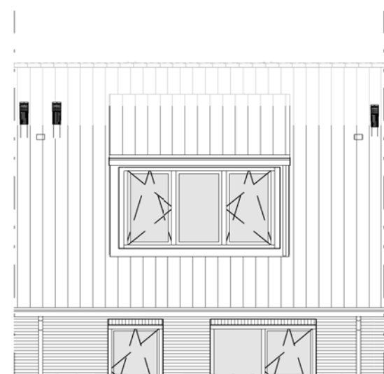
achtergevel - 1 : 100
