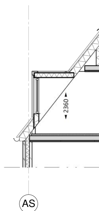
doorsnede 1-1 - 1 : 100
