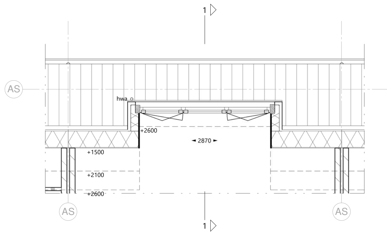
2e verdieping - 1 : 50
