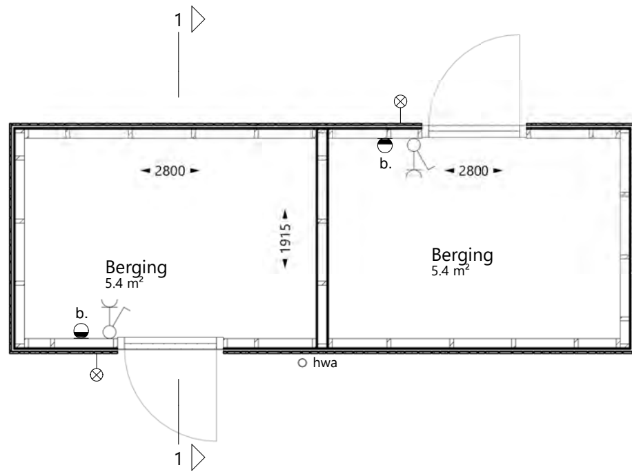
begane grond - 1 : 50
