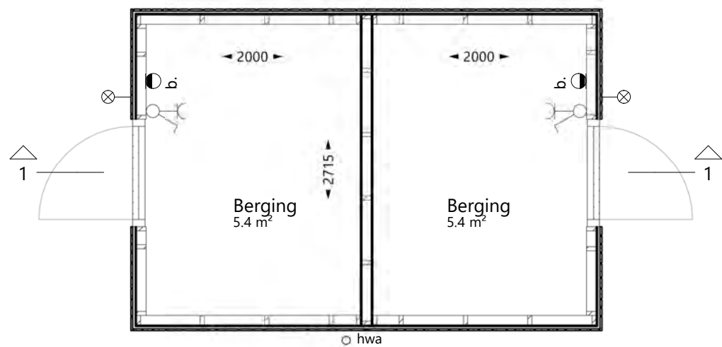
begane grond - 1 : 50
