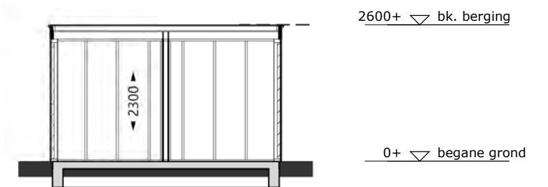
doorsnede 1-1 - 1 : 100
