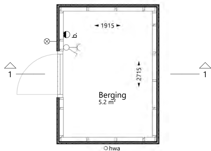
begane grond - 1 : 50
