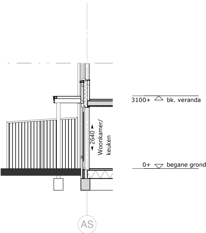
doorsnede 1-1 - 1 : 100
