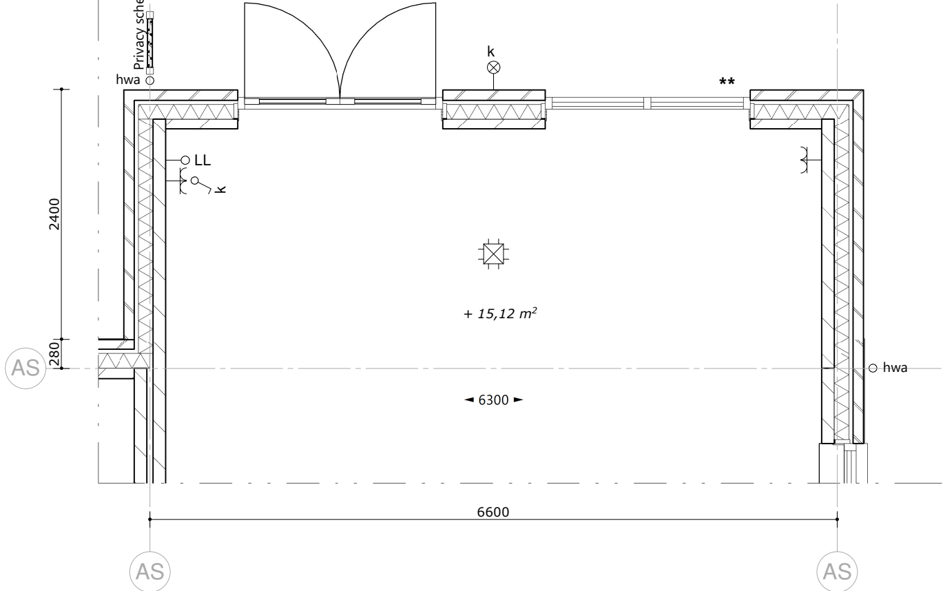
begane grond - 1 : 50
