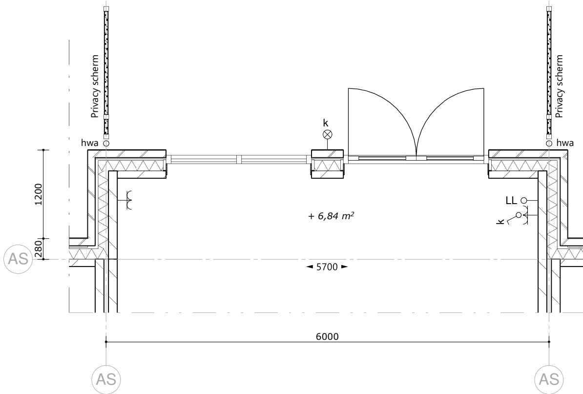
begane grond - 1 : 50
