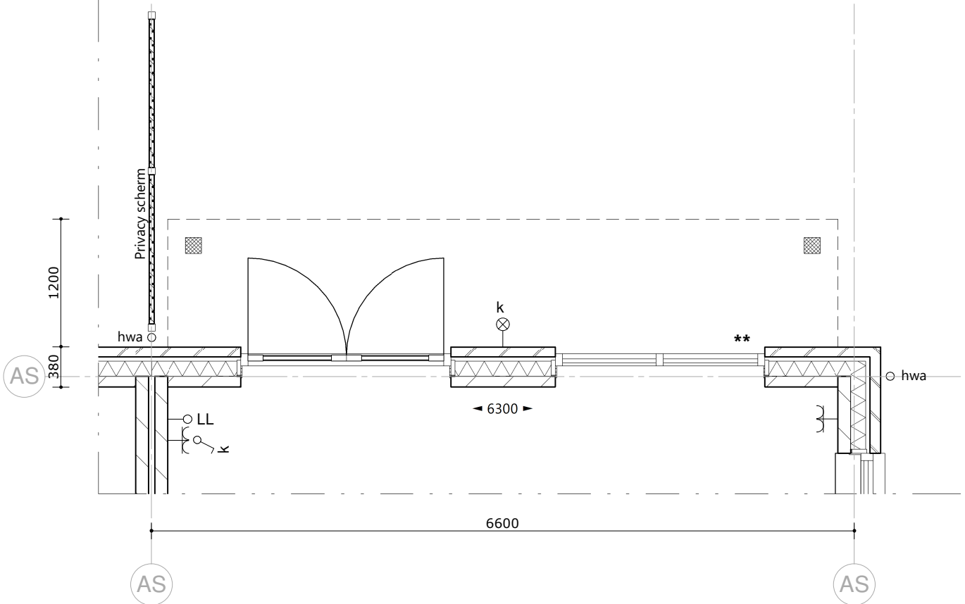
begane grond - 1 : 50
