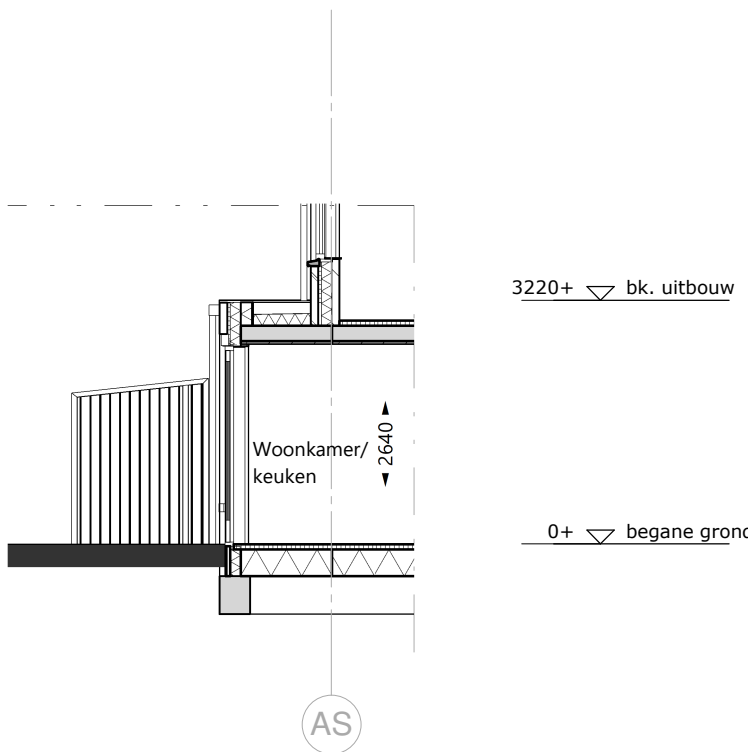
doorsnede 1-1 - 1 : 100
