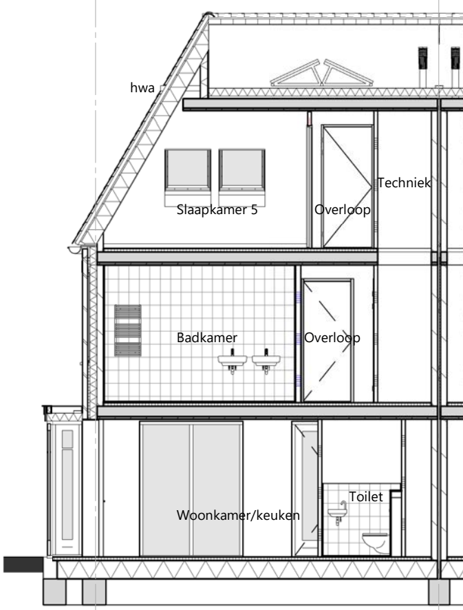
doorsnede A-A - 1 : 100
