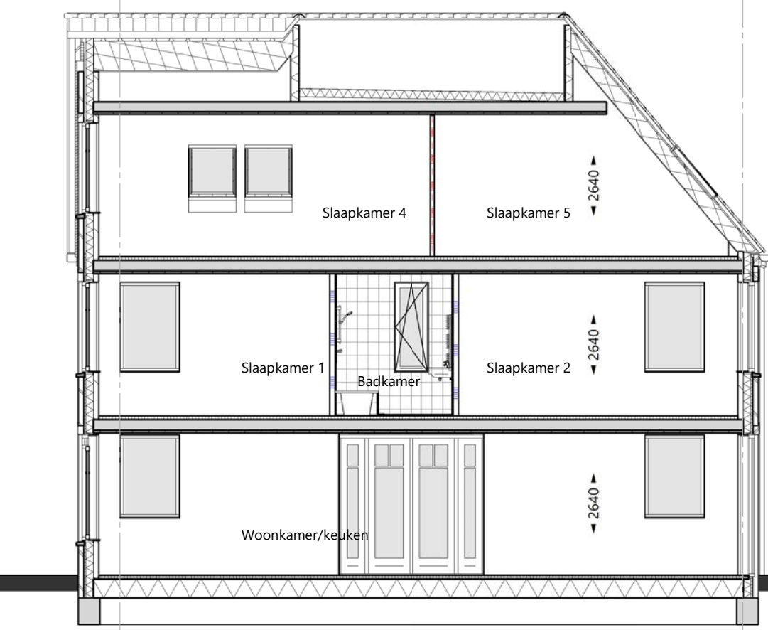
doorsnede 1-1 - 1 : 100
