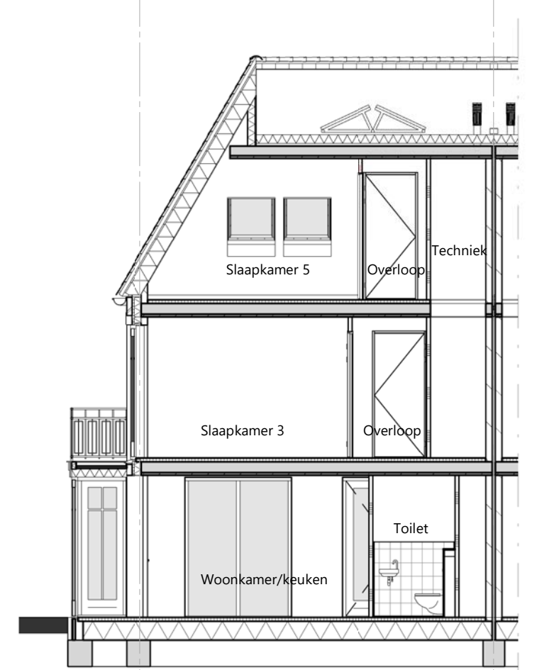
doorsnede A-A - 1 : 100
