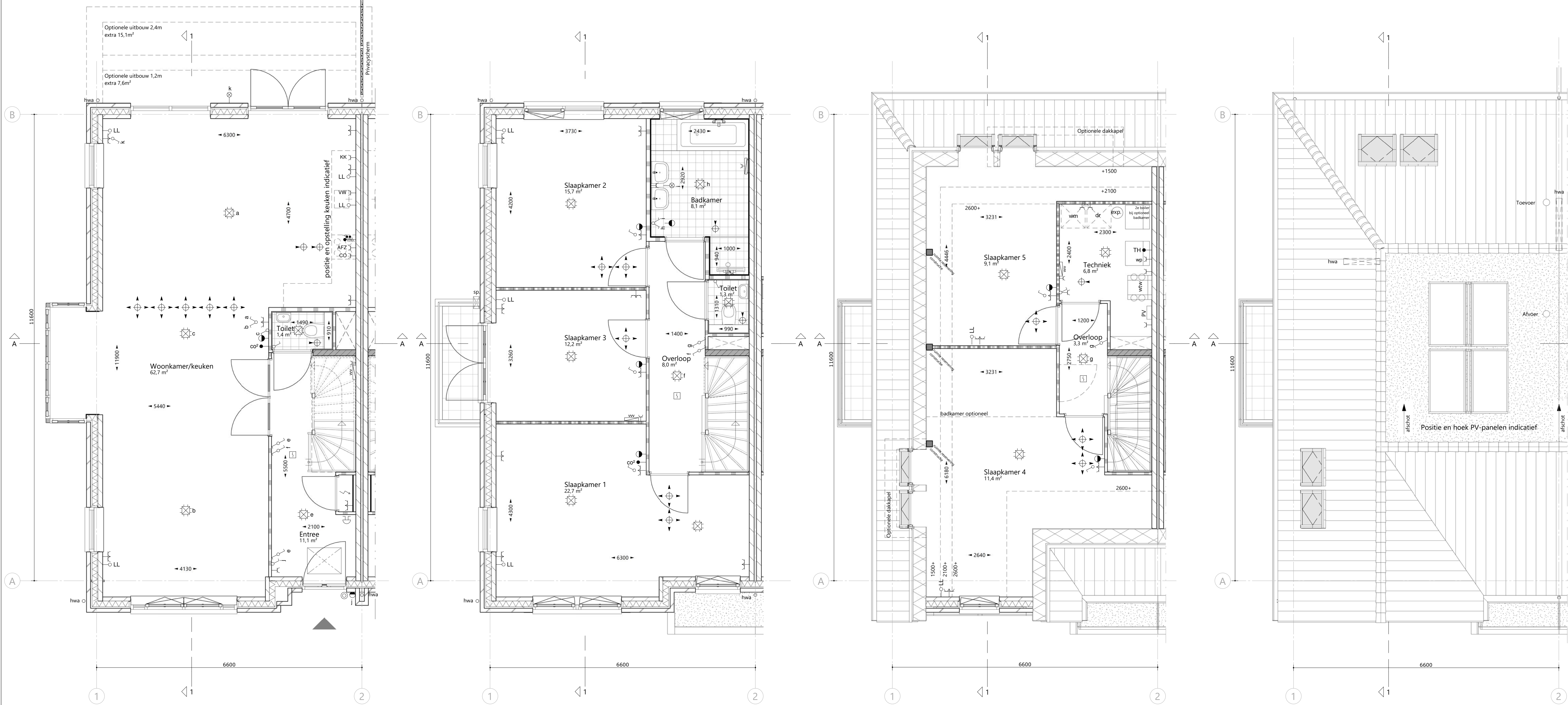
begane grond - 1 : 50 1e verdieping - 1 : 50 2e verdieping - 1 : 50 dakplan - 1 : 50
