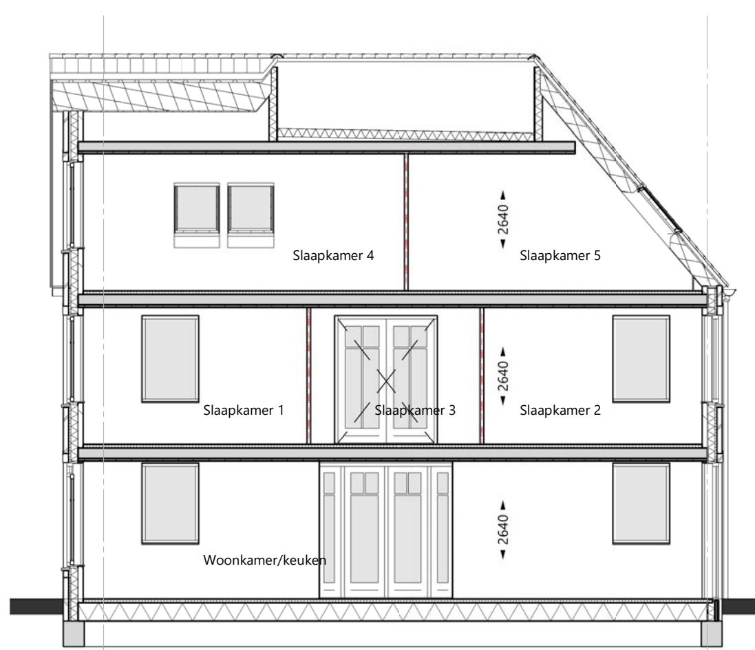
doorsnede 1-1 - 1 : 100
