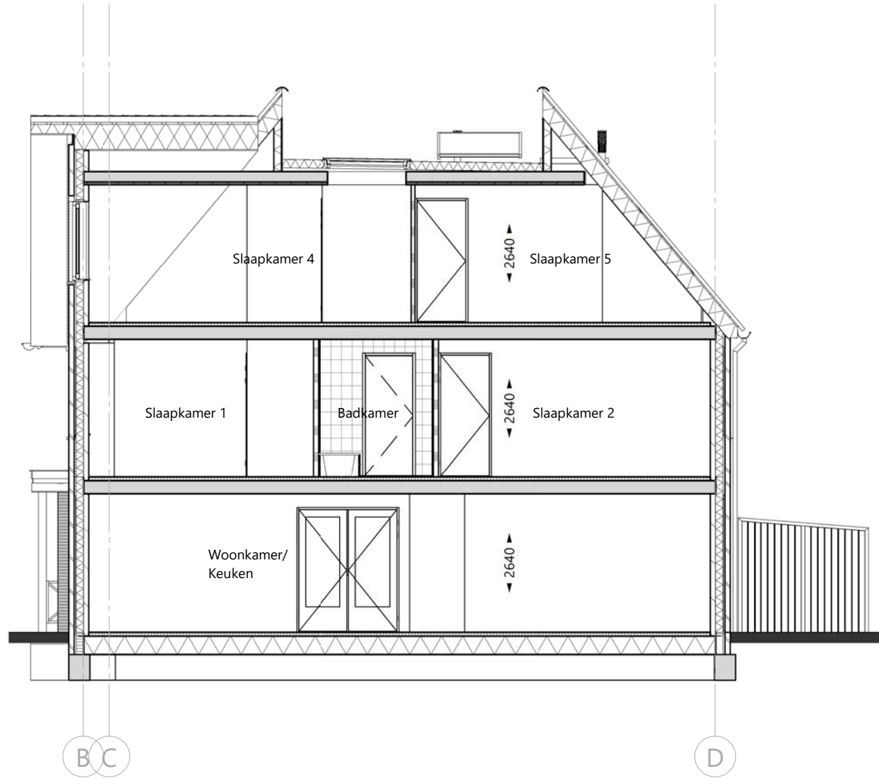
doorsnede 1-1 - 1 : 100
