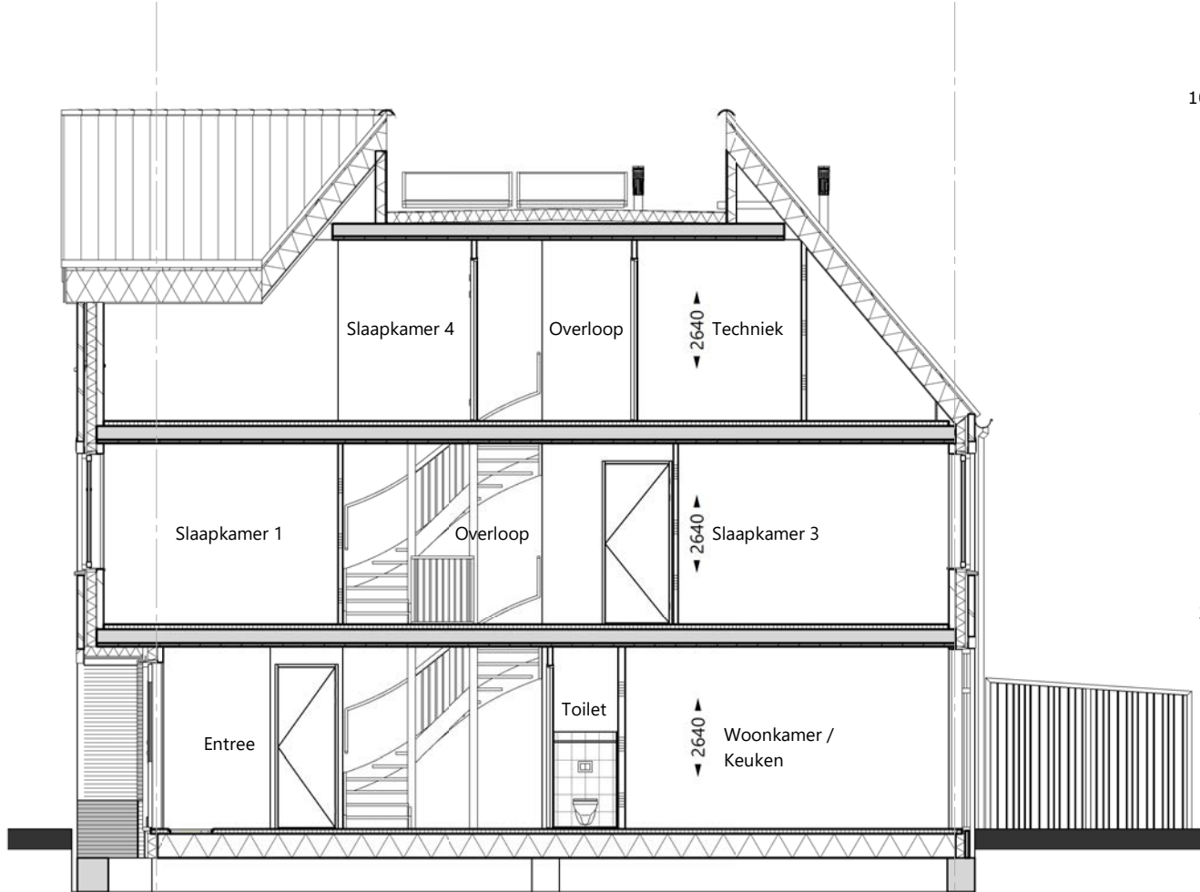
doorsnede 1-1 - 1 : 100
