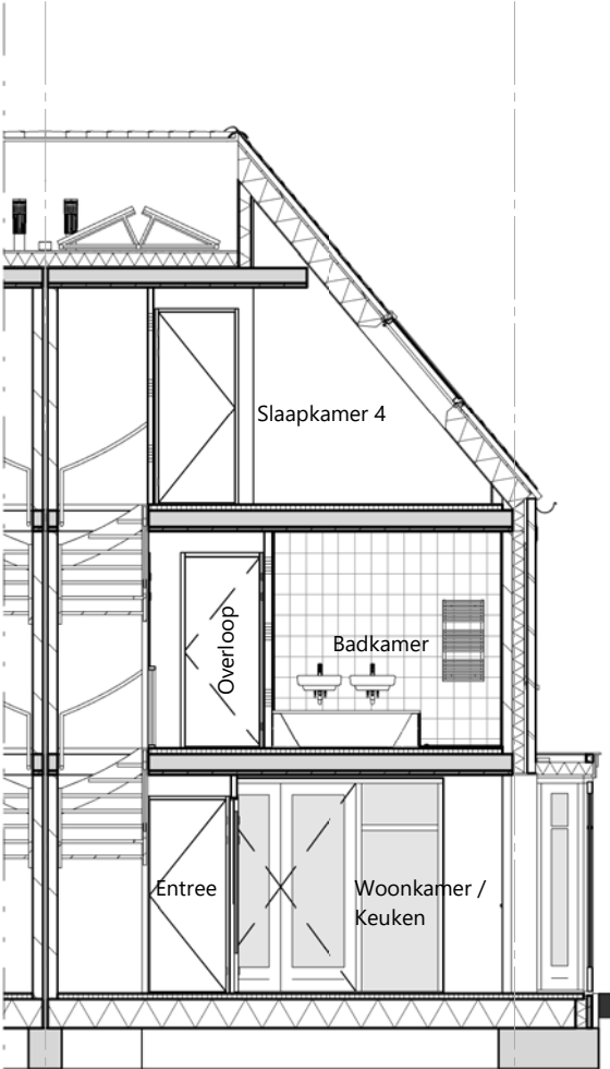
doorsnede A-A - 1 : 100
