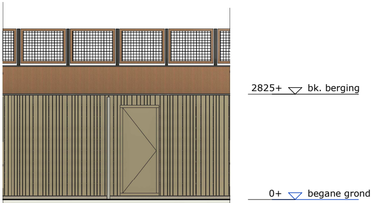
gevelaanzicht - 1 : 100
