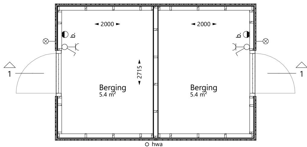
begane grond - 1 : 50
