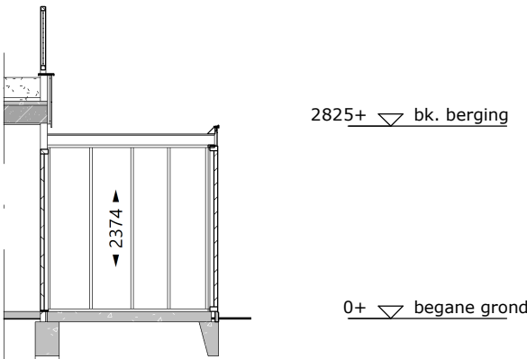
doorsnede 1 - 1 - 1 : 100
