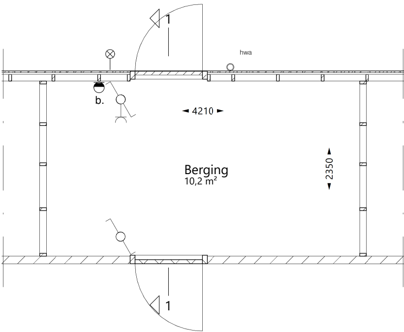
begane grond - 1 : 50
