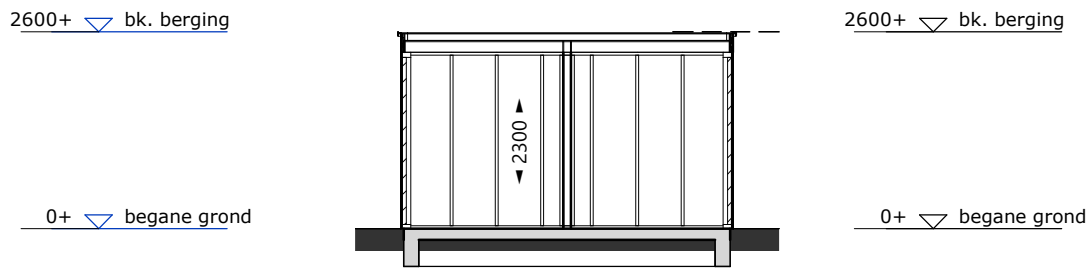
doorsnede 1-1 - 1 : 100
