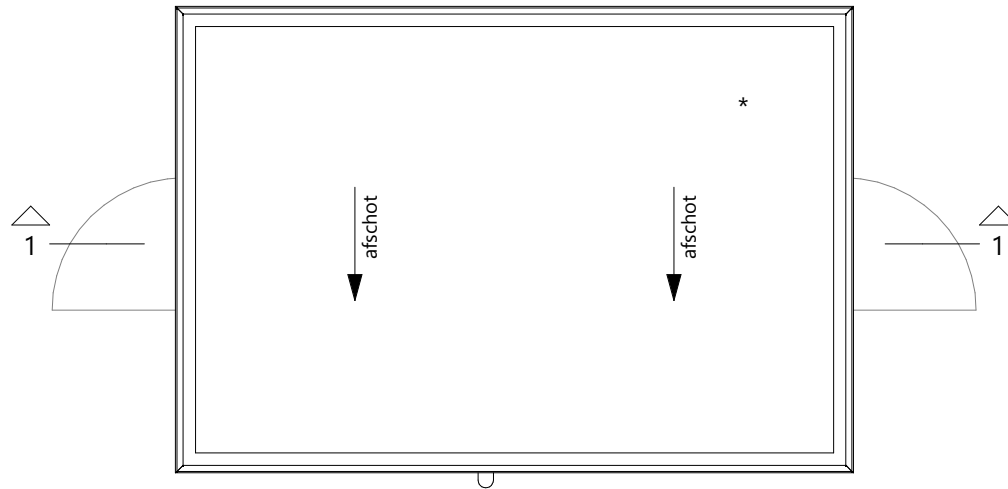
dakaanzicht - 1 : 50
