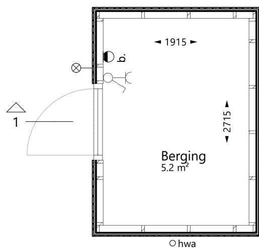
begane grond - 1 : 50
