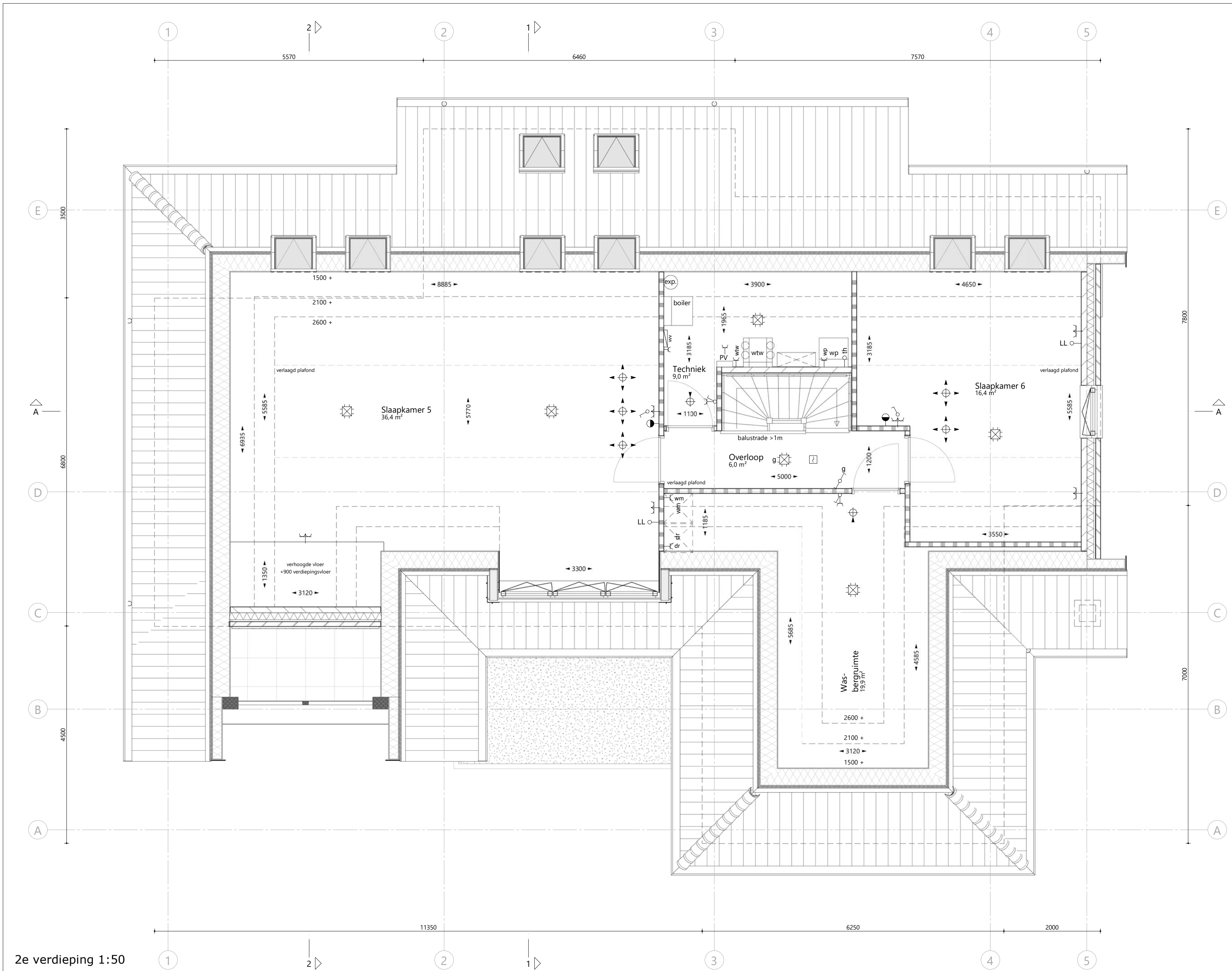
2e verdieping 1:50
