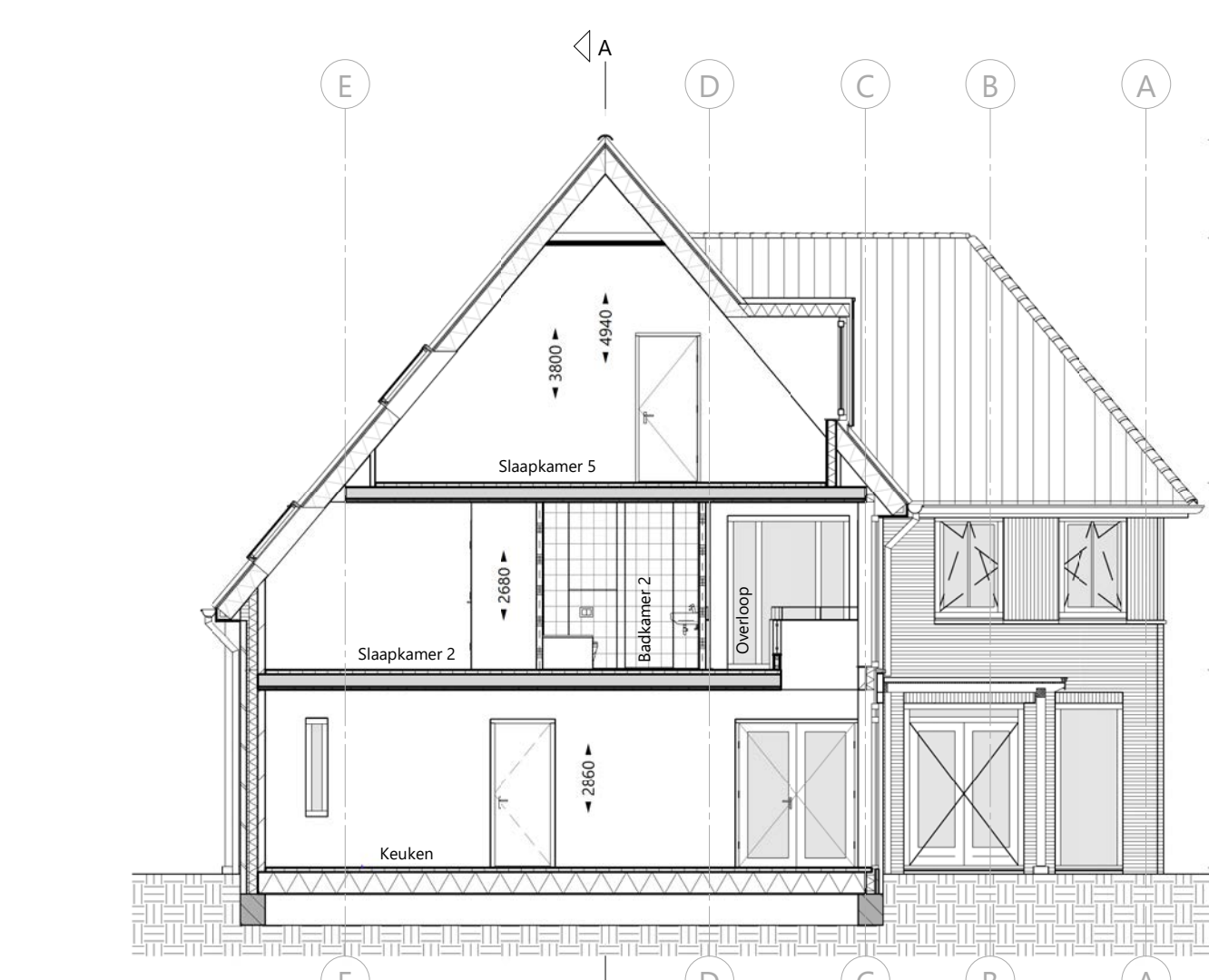
doorsnede 1-1 1:100
