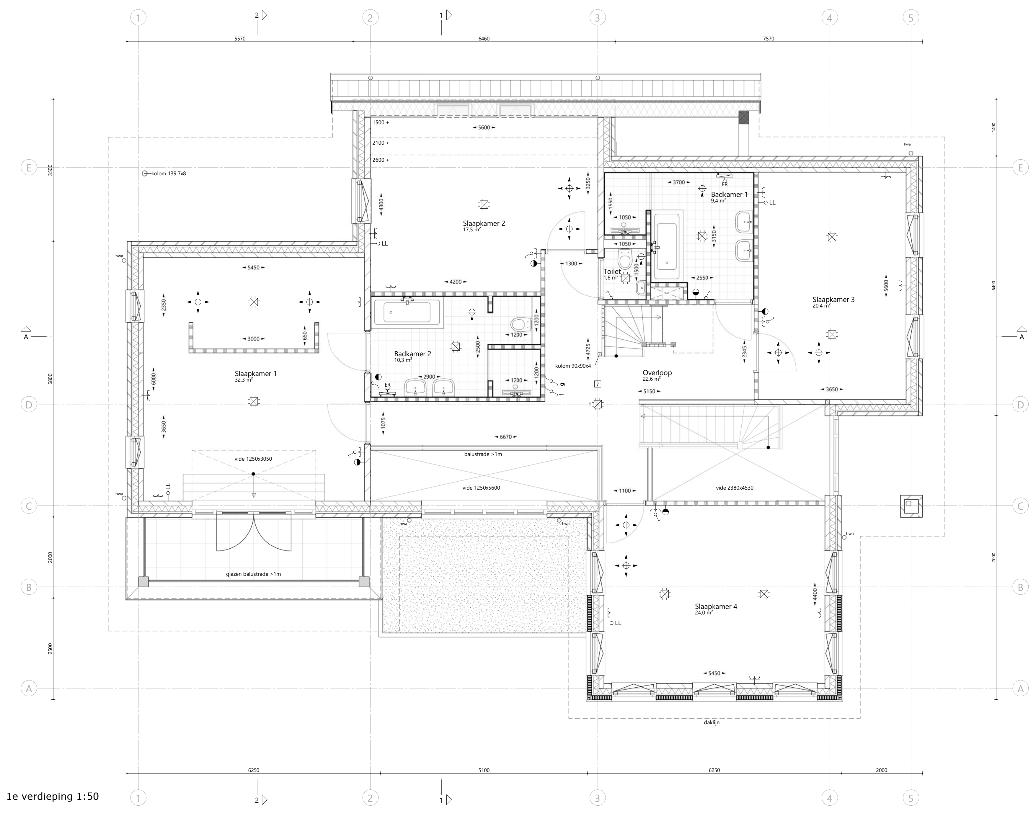
1e verdieping 1:50
