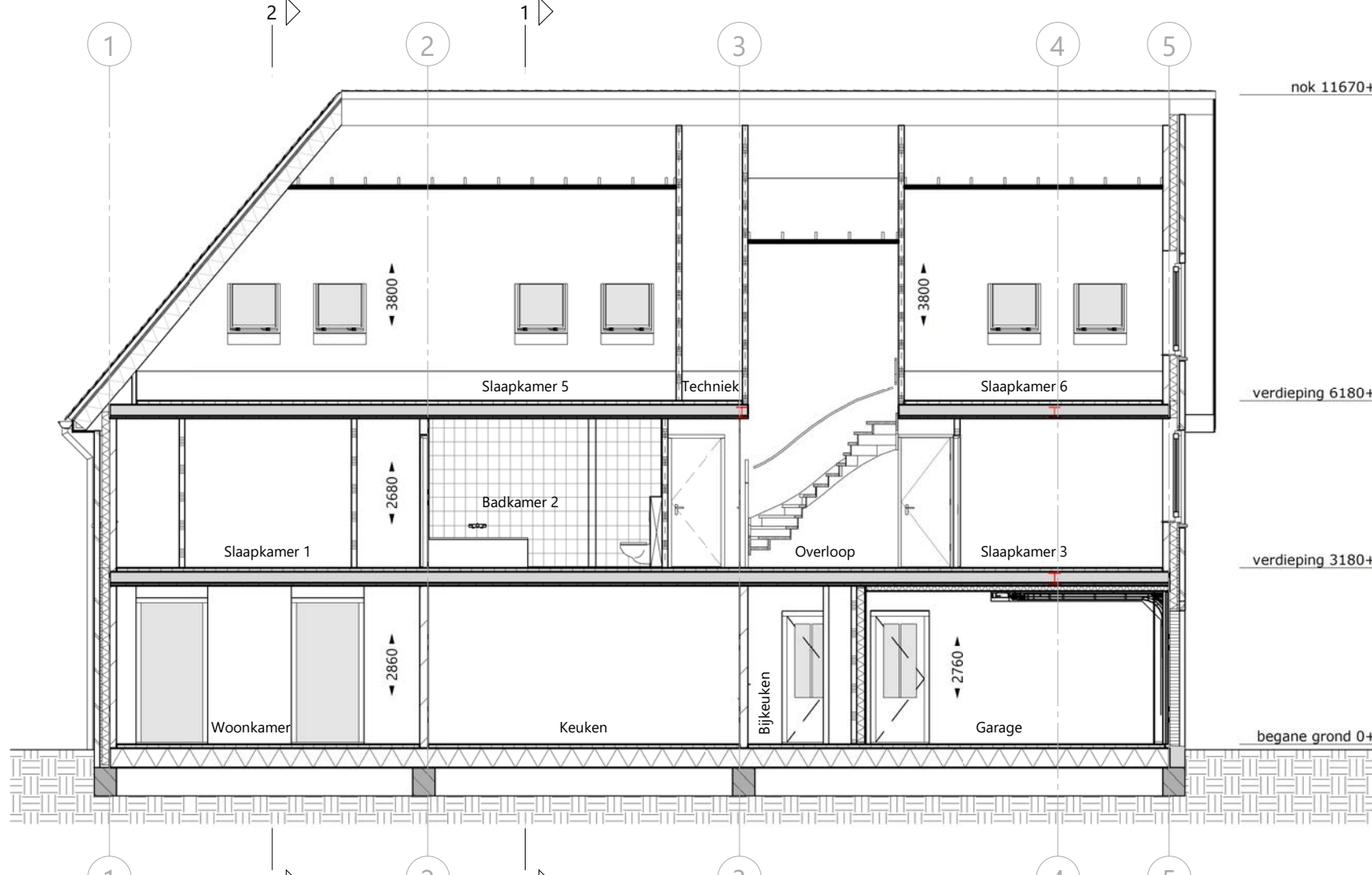
doorsnede A-A 1:100
