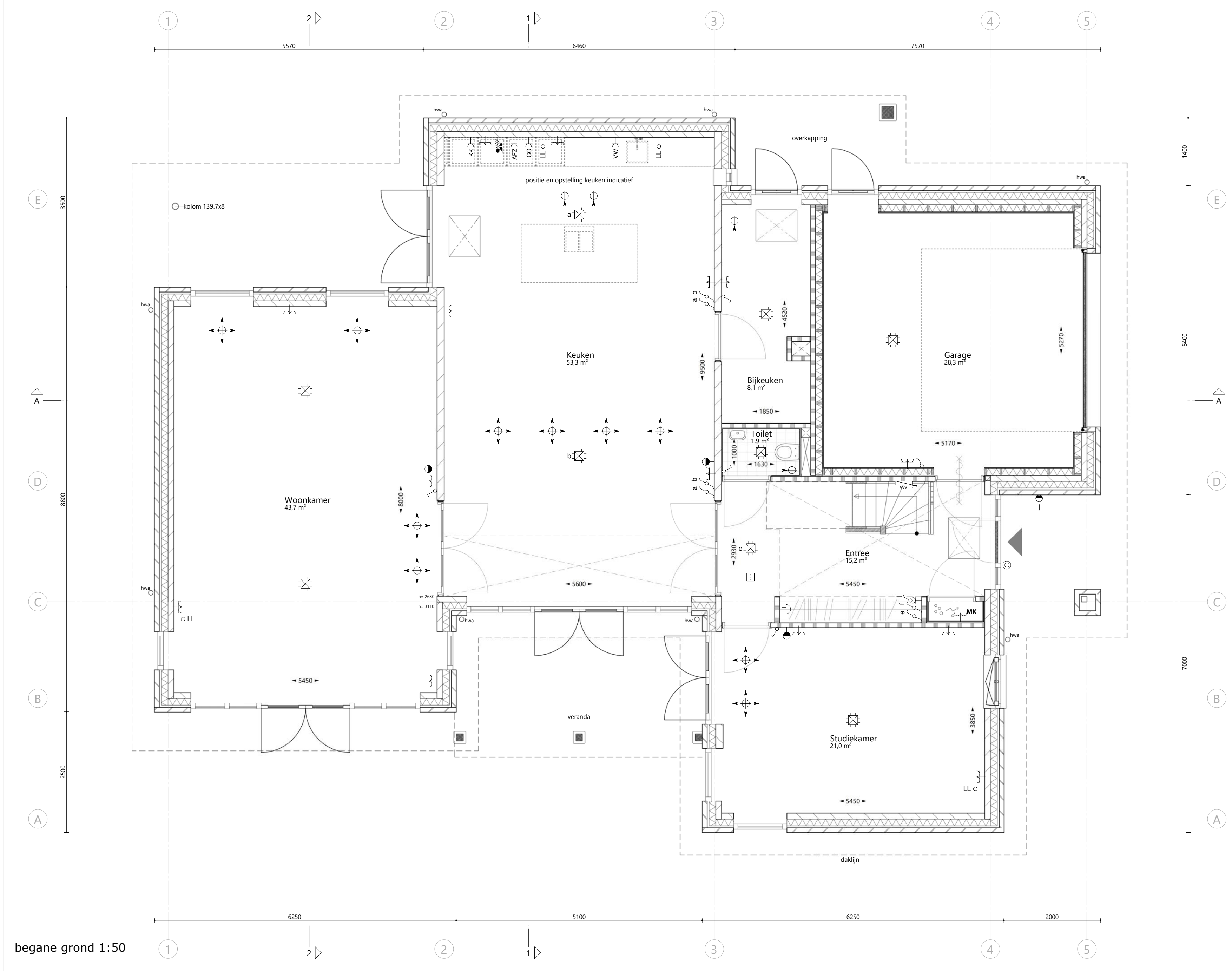
begane grond 1:50
