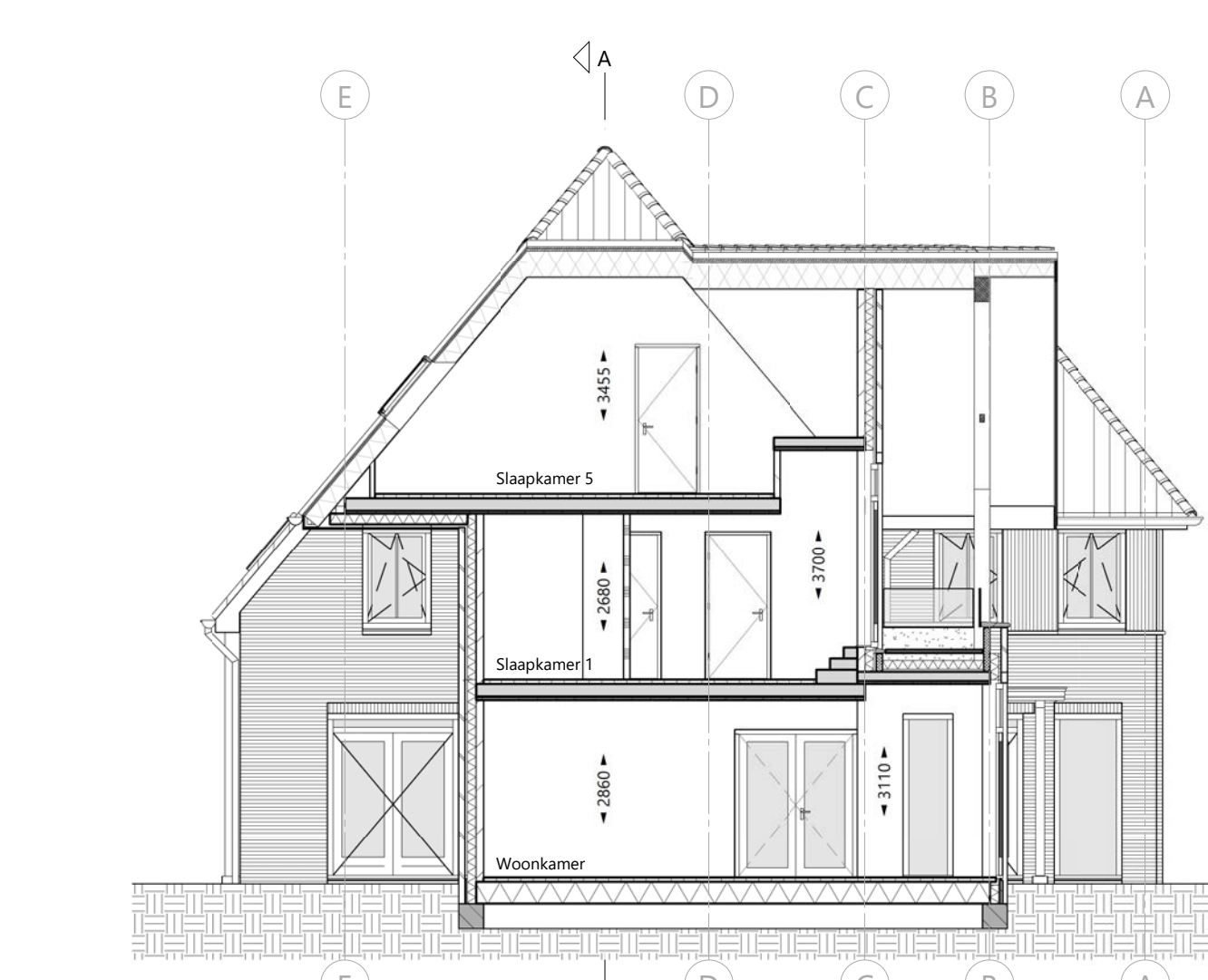
doorsnede 2-2 1:100
