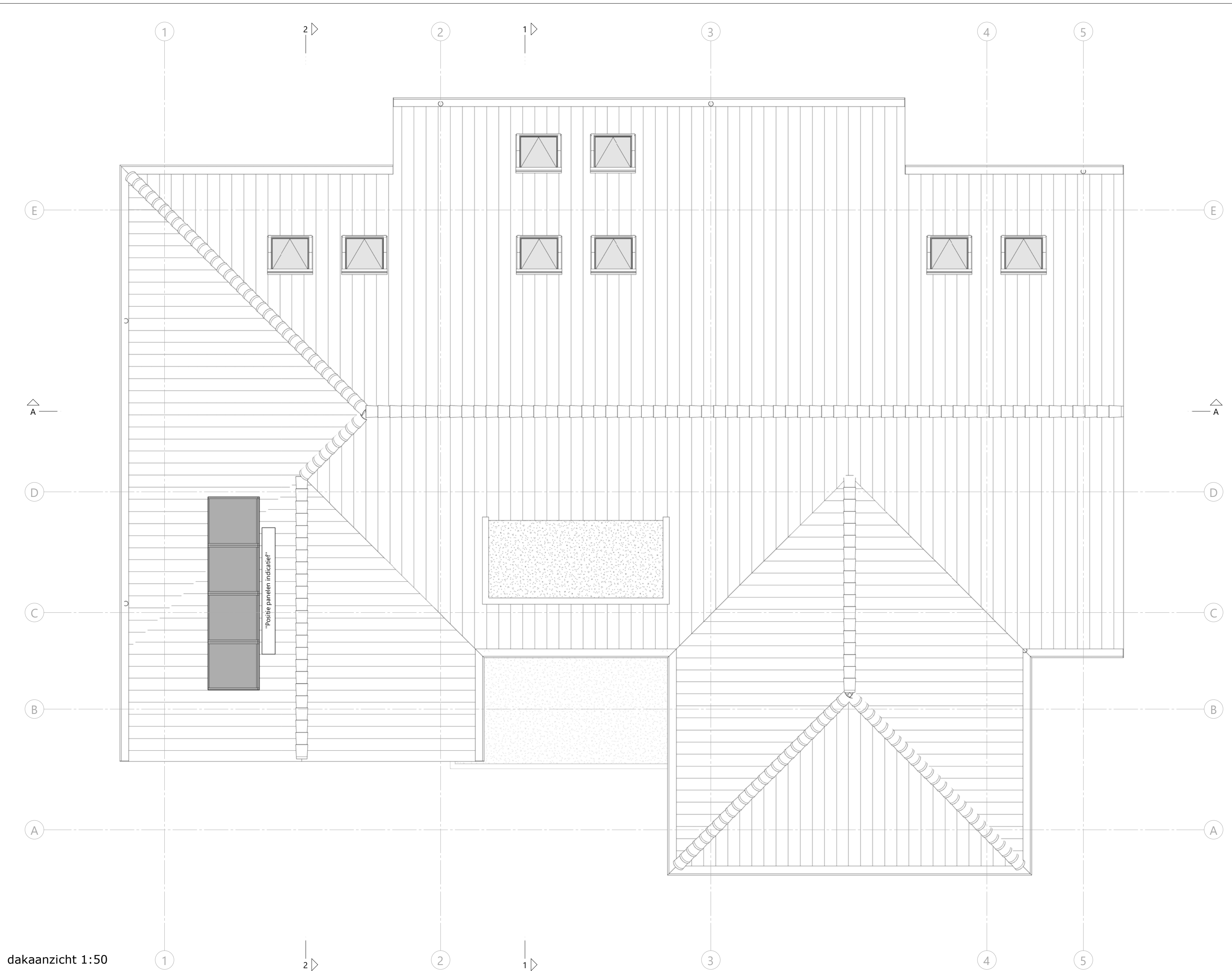
dakaanzicht 1:50
