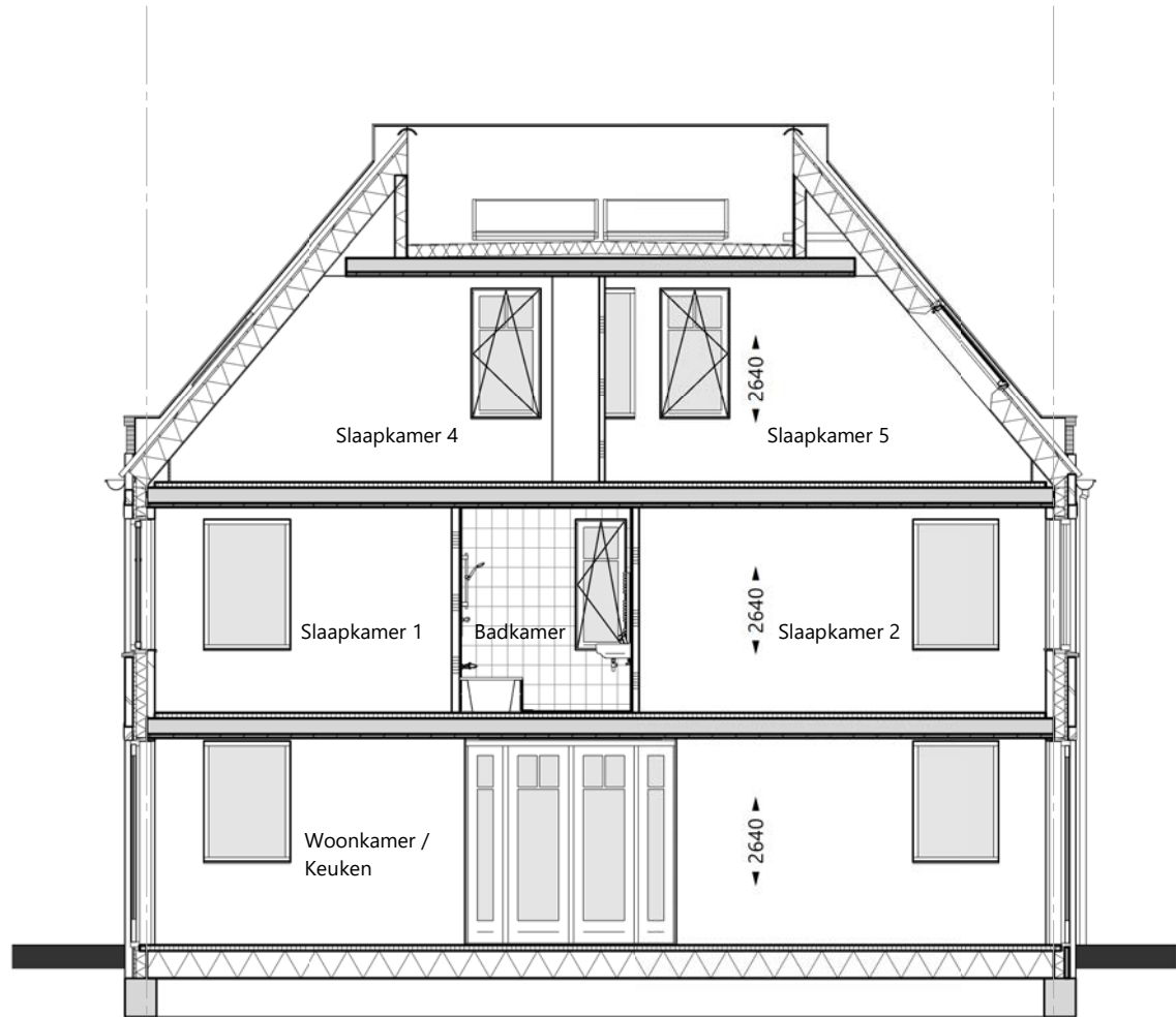
doorsnede 1-1 - 1 : 100
