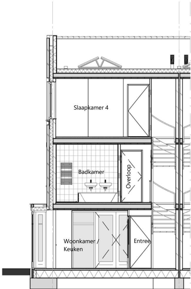
doorsnede A-A - 1 : 100
