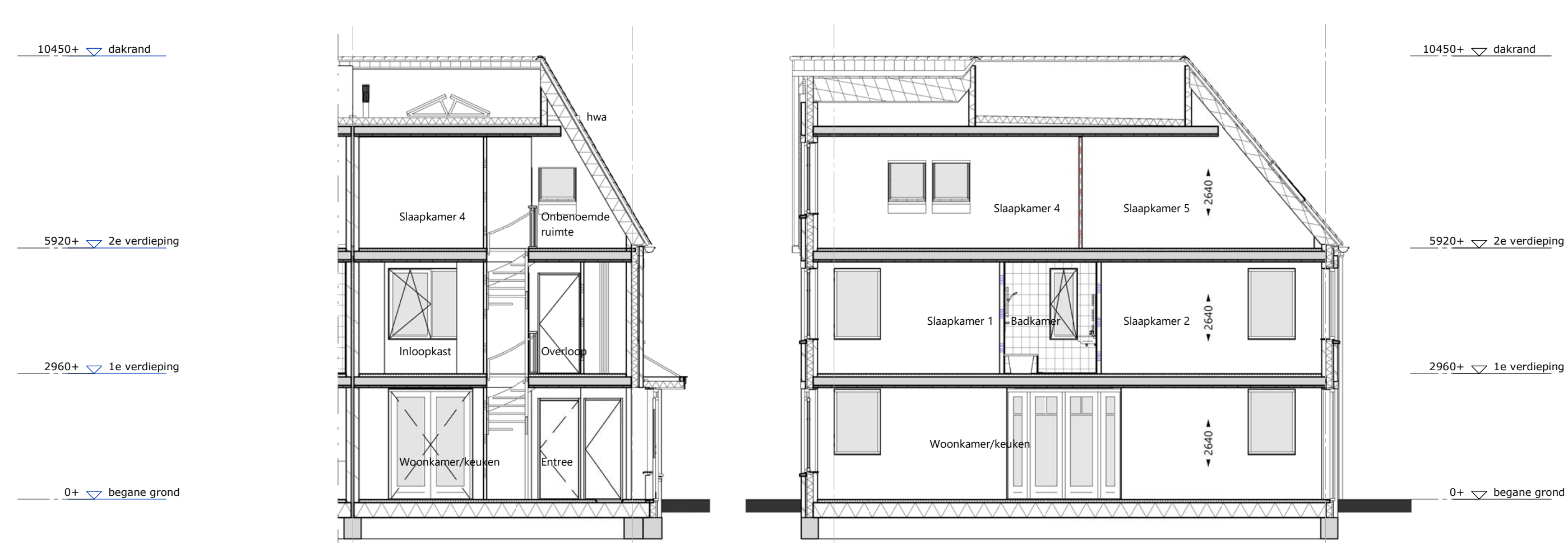
doorsnede A-A - 1 : 100 doorsnede 1-1 - 1 : 100
