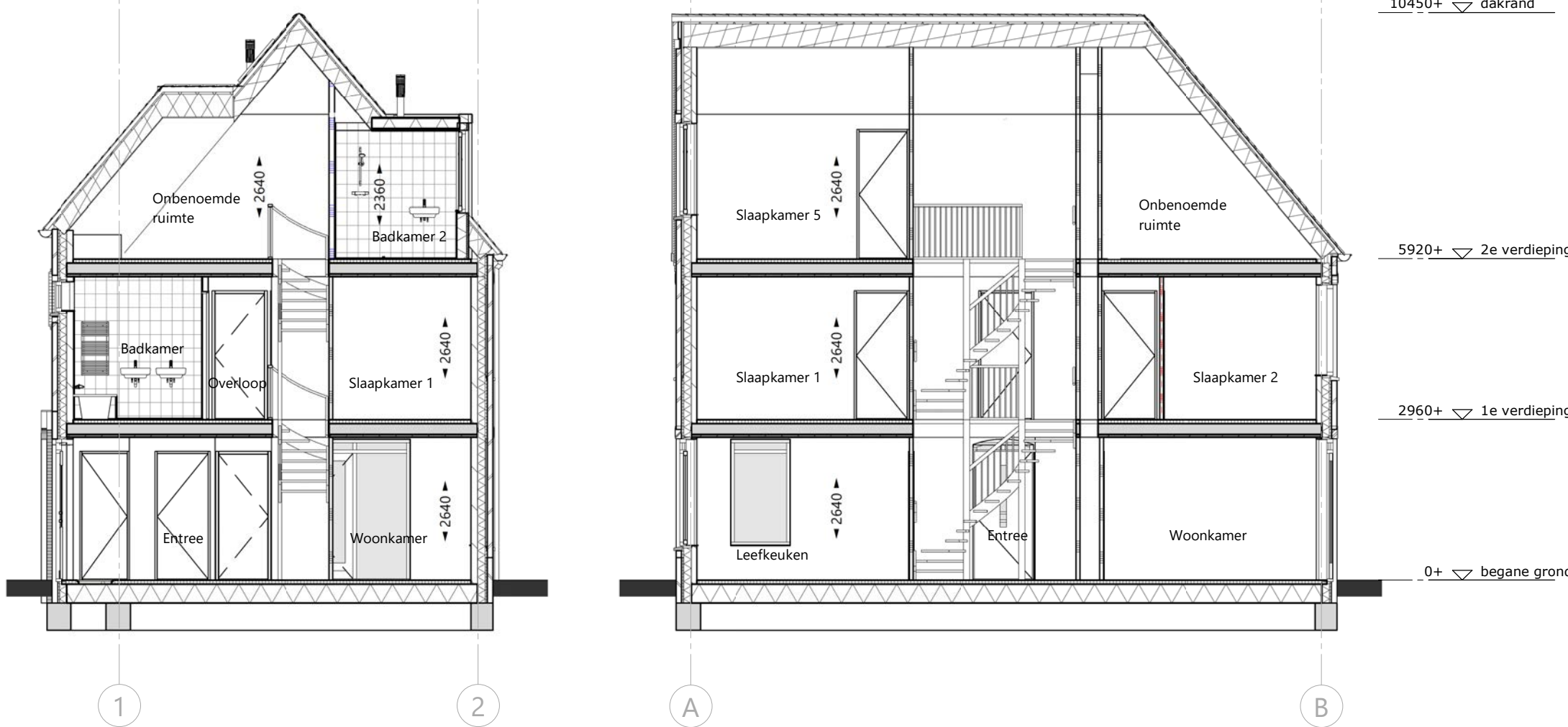
doorsnede A-A - 1 : 100
